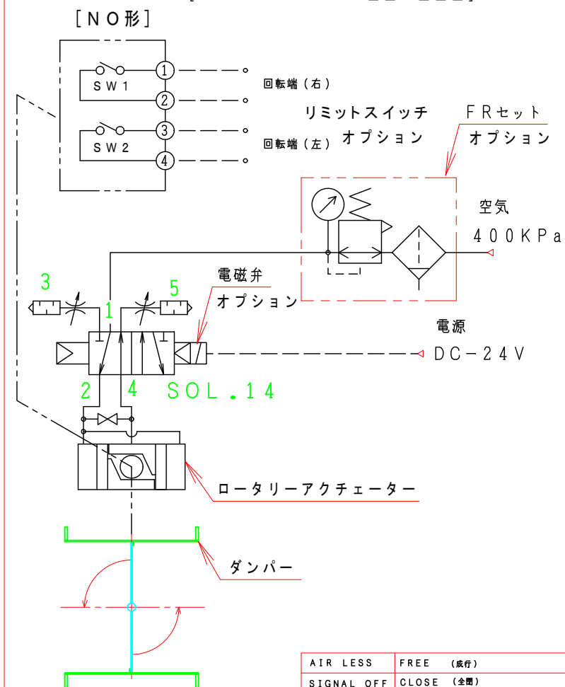
フローシート図
